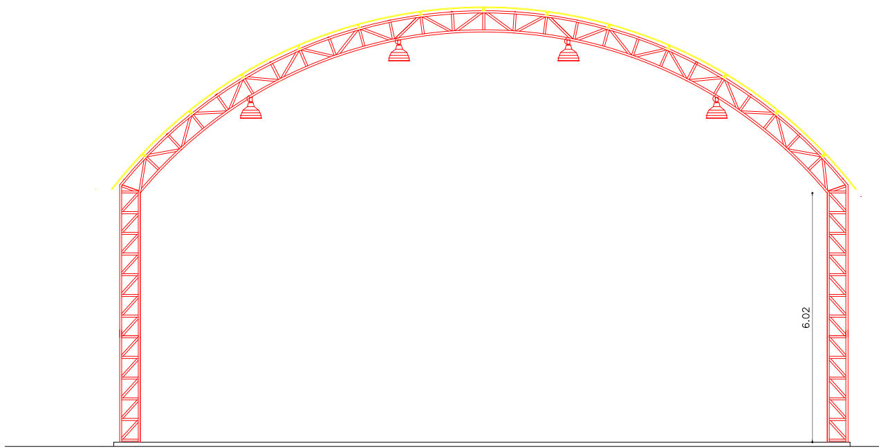
CORTE A.A.
